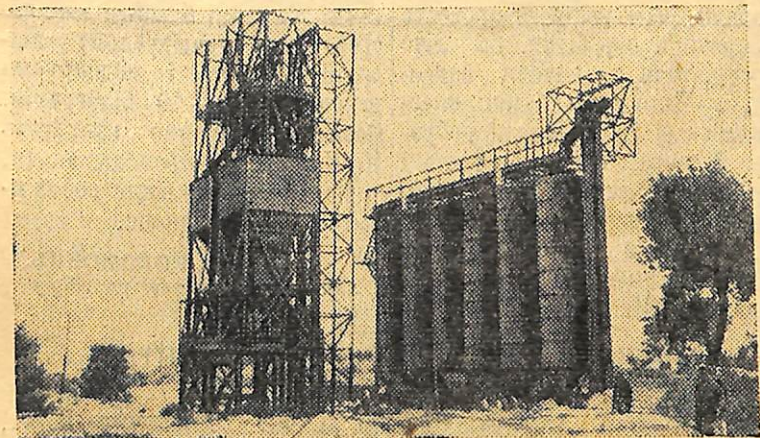
В районі майбутньої Каховської ГЕС до ладу діючих стає все більше підсобних підприємств, призначених для будівництва головних гідротехнічних споруд.
